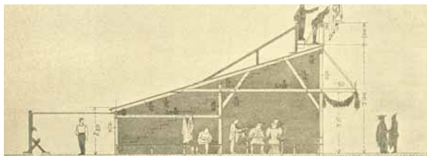
Průřez pobočné tribuny
